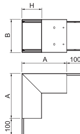
Abmessungen
