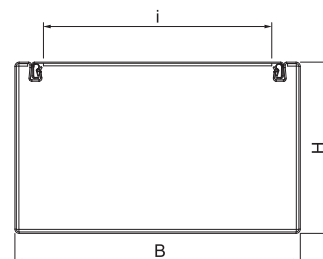
Abmessungen
